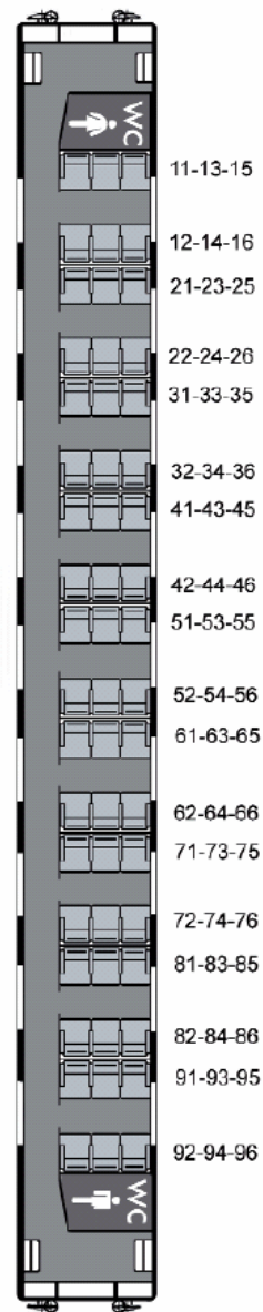
Vettura a scompartimenti 1 a classe
